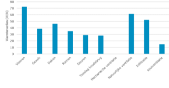
Aandeel warmteverlies, Vrijstaande woningen >1995, Niveau 3
