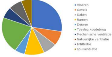
Aandeel warmteverlies, Vrijstaande woningen 1975-1995, Niveau 4
