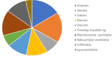
Aandeel warmteverlies, Vrijstaande woningen 1945-1975, Niveau 3
