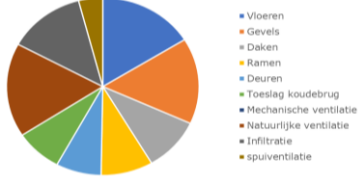
Aandeel warmteverlies, Vrijstaande woningen 1975-1995, Niveau 3
