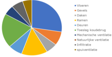
Aandeel warmteverlies, Vrijstaande woningen 1945-1975, Niveau 4
