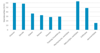
Aandeel warmteverlies, Vrijstaande woningen 1975-1995, Niveau 3
