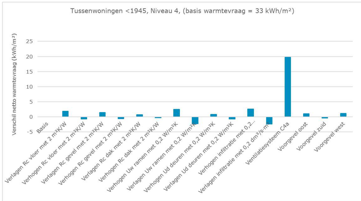
Figuur 22: gevoeligheidsanalyse tussenwoning, basisuitgangspunten tussenwoning (niveau 4, tussenwoning < 1945)
