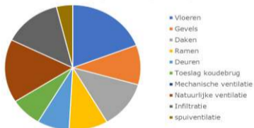
Aandeel warmteverlies, Vrijstaande woningen >1995, Niveau 3
