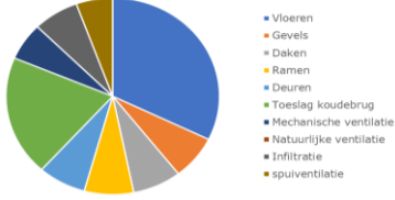
Aandeel warmteverlies, Vrijstaande woningen <1945, Niveau 4
