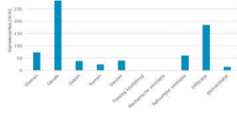
Aandeel warmteverlies, Vrijstaande woningen <1945, Niveau 3
