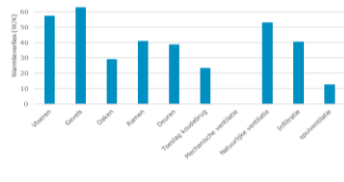
Aandeel warmteverlies, Vrijstaande woningen 1945-1975, Niveau 3
