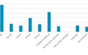
Aandeel warmteverlies, Vrijstaande woningen 1945-1975, Niveau 4
