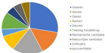
Aandeel warmteverlies, Vrijstaande woningen >1995, Niveau 4
