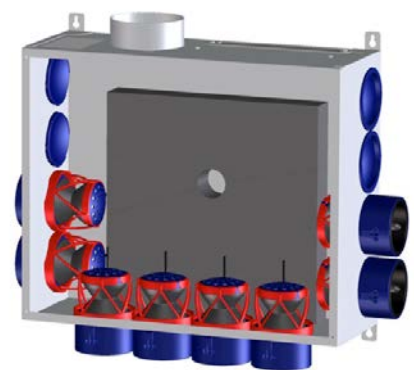
Een verdeelbox (plenum) met regelbare kleppen. Ieder afvoerpunt is met een apart ventilatiekanaal hierop aangesloten. Met de kleppen wordt de capaciteit per afvoerpunt geregeld.
