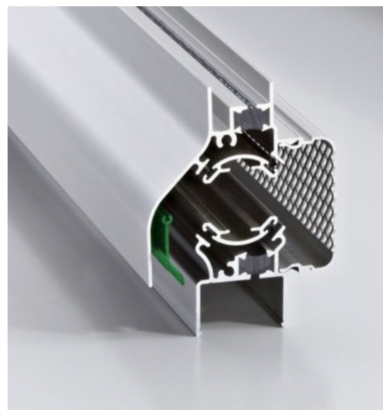
Eenvoudig zelfregelend ventilatierooster. Bij winddruk sluit het groene flapje de instroomopening meer of minder af. De bewoner kan het afdekrooster eraf nemen om het geheel schoon te maken.
