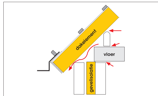
Figuur 1: Overall waar de thermische lijn wordt doorbroken zijn koudebruggen aanwezig, ofwel plekken met een warmteweerstand die lager is dan aangrenzende delen. Dit zijn ook potentiële luchtlekken.
